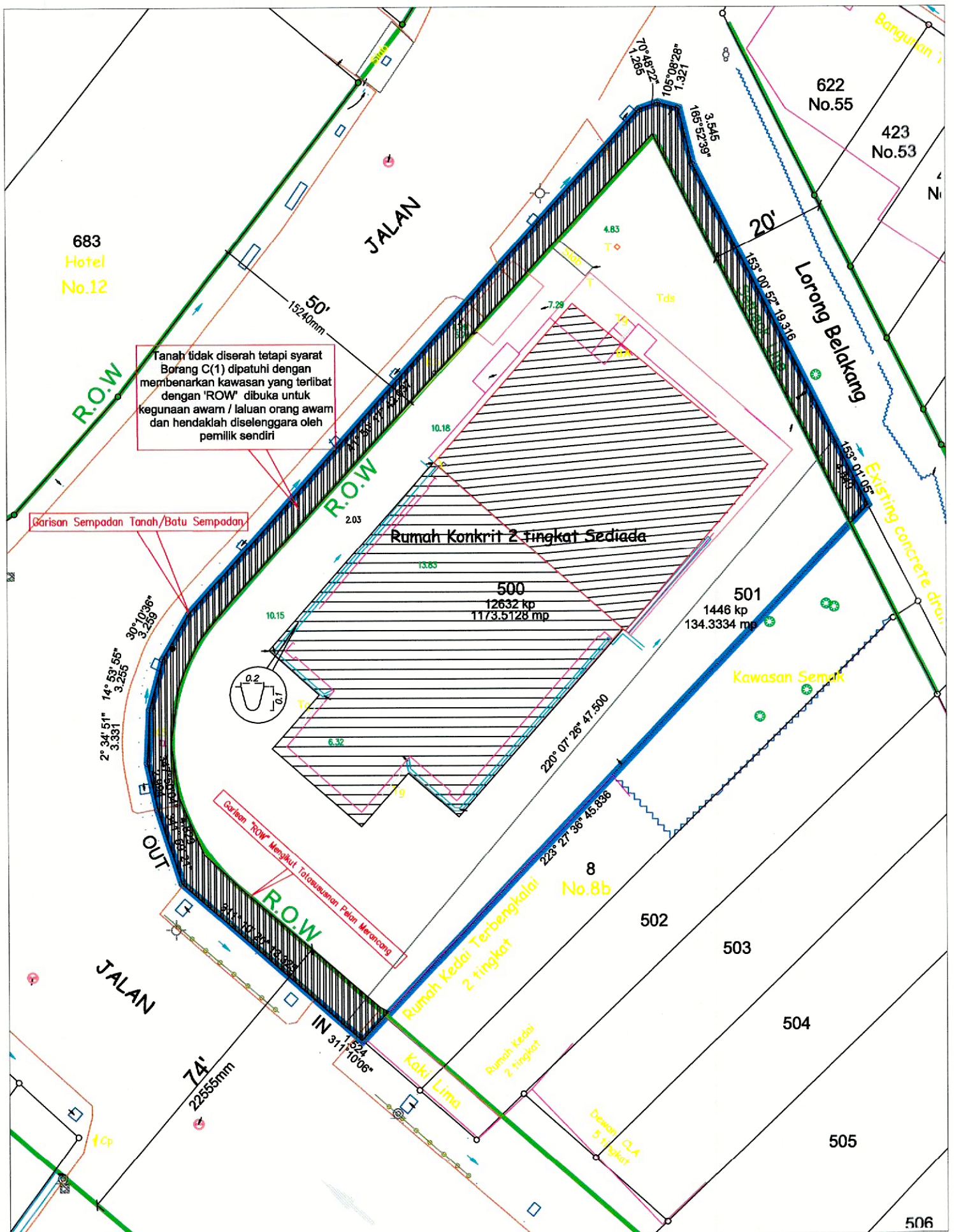
Contoh Senario Garis Panduan Perkara 3 : Pelan Permohonan Kebenaran Merancang Bagi Syarat Penyerahan Tanah Dikecualikan Tetapi Syarat Tambahan Diletakkan Dalam Borang C(1)
